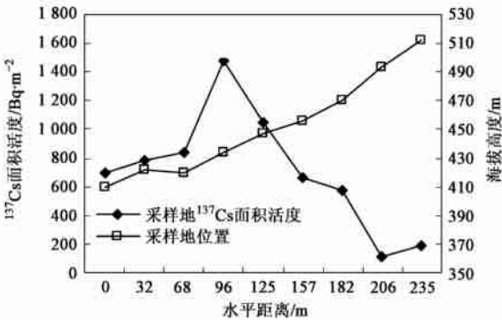
图 4 耕地坡面采样地位置及样地 137 Cs 面积活度
