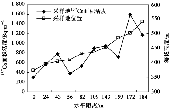
图 2 次生林坡面采样地位置及样地 137 Cs 面积活度
