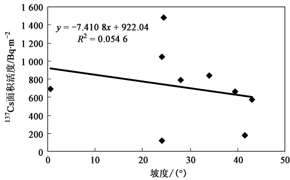
图5 农耕地 137 Cs面积活度与坡度的关系
