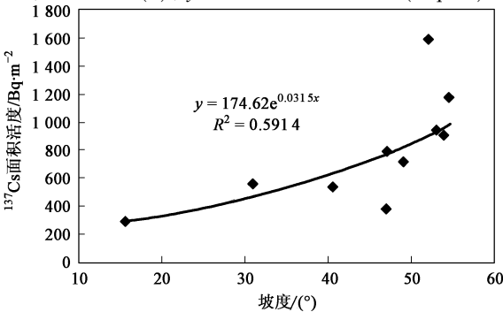
图 3 次生林地 137 Cs 面积活度与坡度的关系
