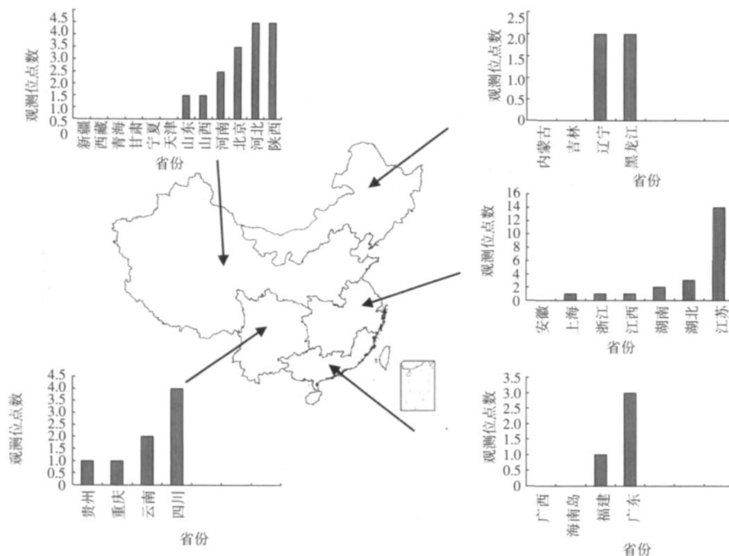
图 2 农田 N_2O 通量观测位点的区域分布
