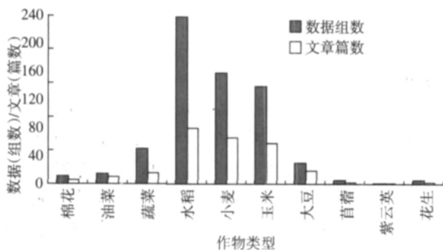
图 3 农田 N_2O 通量观测在不同作物间的分布
