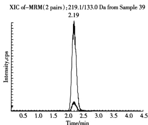
图 1 NP 标准物的提取离子色谱图
