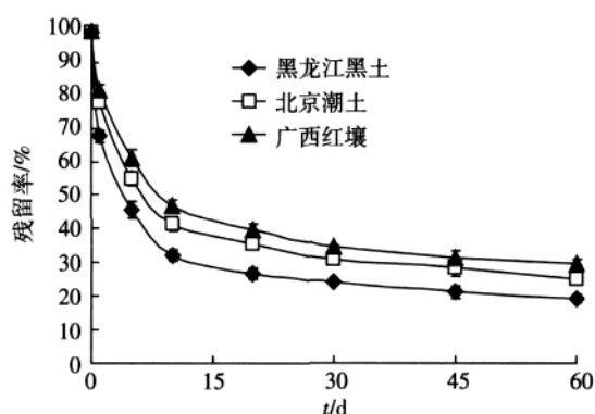
图 2 土壤中 NP 的降解残留率
