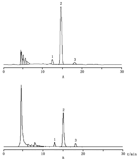
图 1 混合对照品 (A) 和样品 (B) 色谱图
