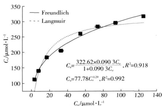
图 3 诺氟沙星在胡敏酸上的吸附等温线
