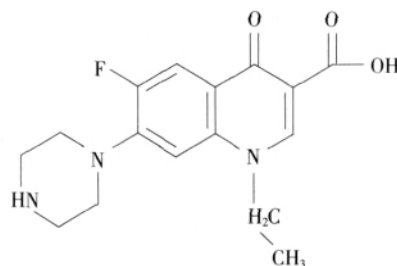
图 1 诺氟沙星的分子结构
