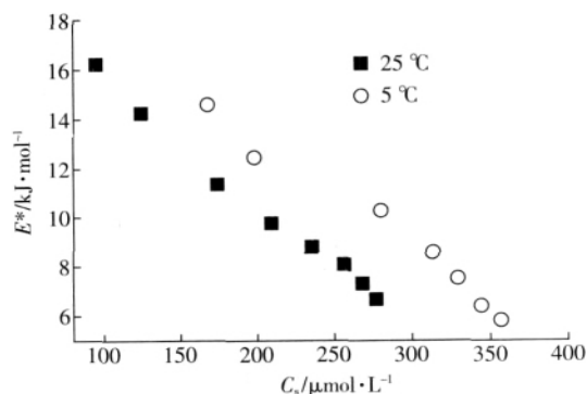
图 5 吸附量和 E^* 的关系
