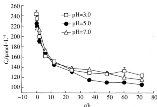
图2 诺氟沙星在胡敏酸上的吸附动力学曲线 Figure 2 Sorption kinetics of Nor on the humic acid
