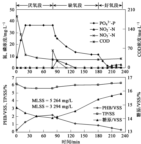
图 6 反应器运行 653 d 时 1 个周期内各参数变化
