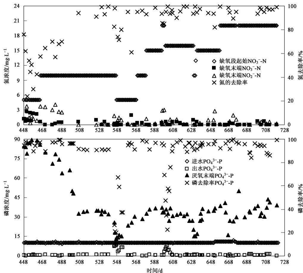
图 5 反硝化聚磷颗粒污泥试验期间氮和磷的历时变化
