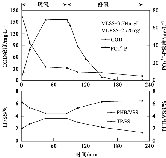
图4 反应器运行第437 d 1个周期内各参数变化
