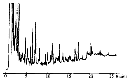
图 11 香附(伪品麦冬)裂解气相色谱图
