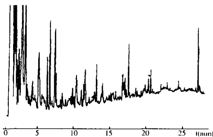
图 8 苍术裂解气相色谱图
