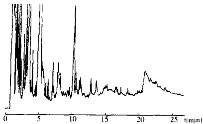
图 9 湖北麦冬裂解气相色谱图
