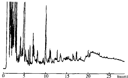
图 10 浙江萧山麦冬裂解气相色谱图
