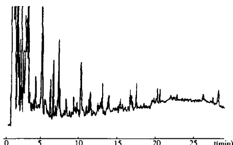
图 7 白术裂解气相色谱图
