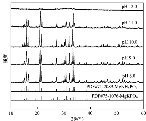
图4 不同 pH 条件下沉淀物的 XRD 谱图
