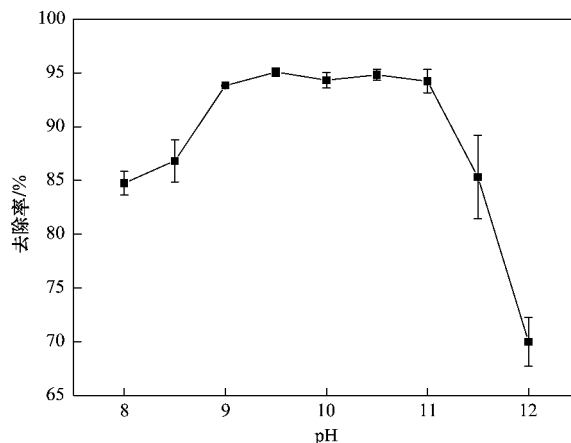
图 1 不同 pH 条件下 \text{PO}_4^{3-}-\text{P} 的去除率
