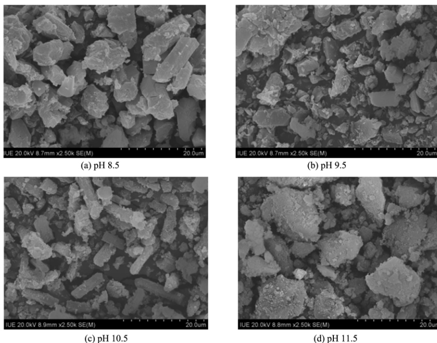
图 2 不同 pH 条件下沉淀物的 SEM 图
