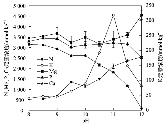
图5 不同 pH 条件下沉淀物元素分析
