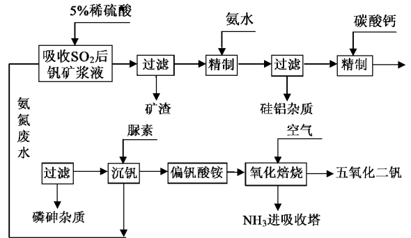
图 6 五氧化二钒提取工艺流程示意
