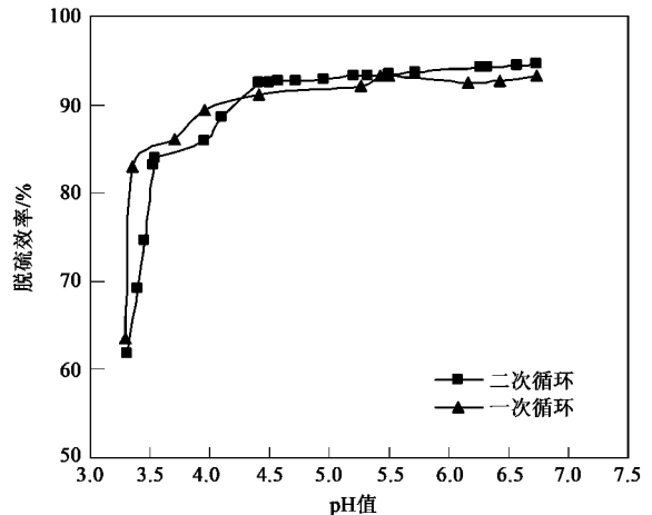
图4 吸收剂循环次数对脱硫效率的影响
