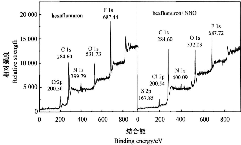
图 4 吸附 NNO 前后的氟铃脲 XPS 电子能谱图
