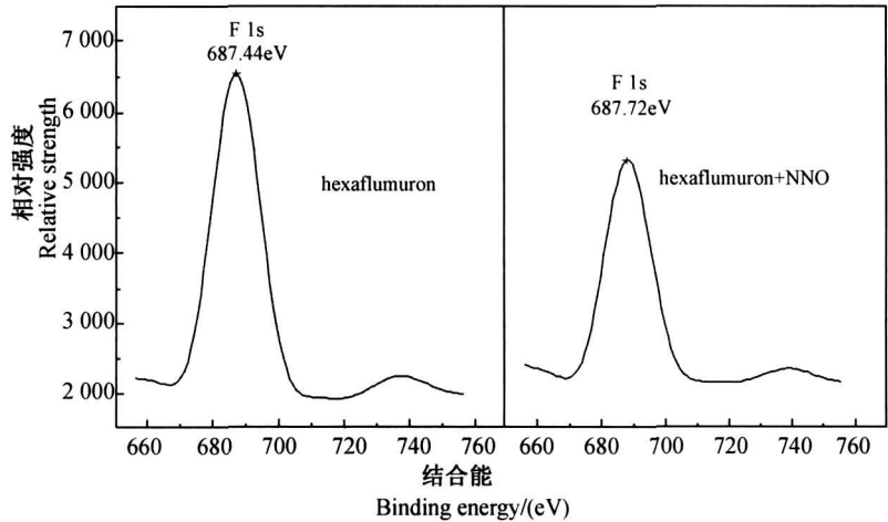
图 5 吸附 NNO 前后的氟铃脲 F1s 的 XPS 电子能谱图
