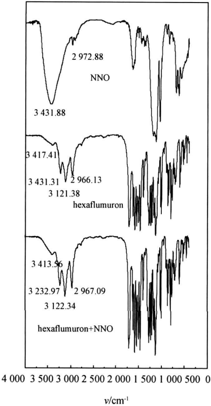
图 1 吸附 NNO 前后的氟铃脲红外光谱图
