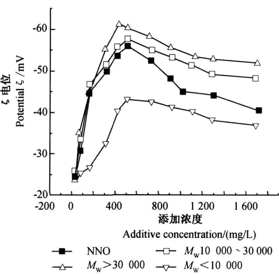
图 3 NNO 质量分数对 \zeta 电位的影响
