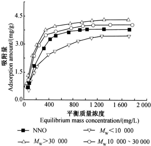
图 2 不同分子质量分散剂在氟铃脲表面的吸附等温线
