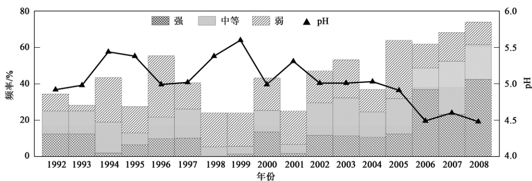
图 3 合肥市各级酸雨发生频率及年均降水 pH 值演变趋势
