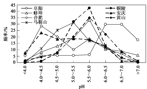
图 1 2006~2008 年各县 pH 值分布
