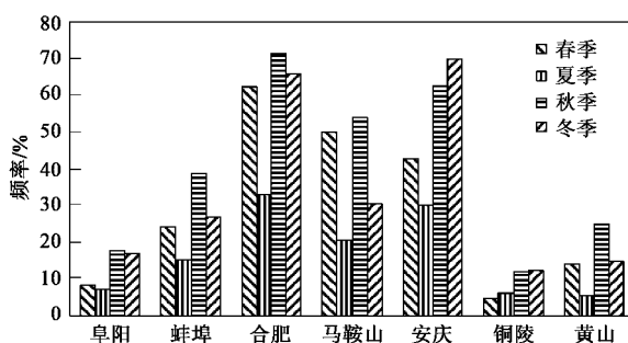
图 2 2006~2008 年安徽各测站中度以上酸雨发生频率的季节分布
