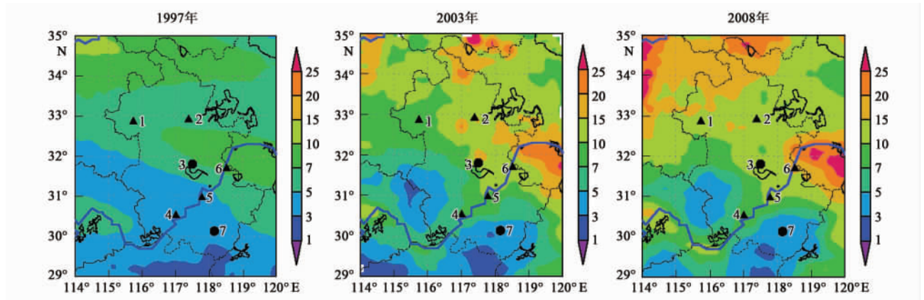
1. 阜阳 2. 蚌埠 3. 合肥 4. 安庆 5. 铜陵 6. 马鞍山 7. 黄山; 单位: 10^{15} 分子 \cdot \text{cm}^{-2} ; GOME:1997; SCIAMACHY:2003, 2008
