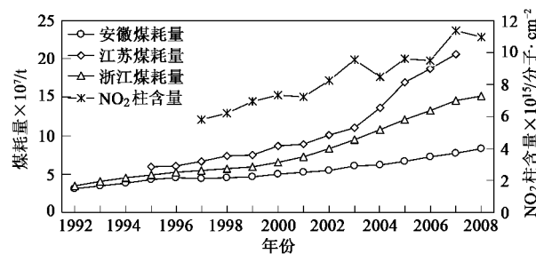
图5 安徽、浙江和江苏煤耗量与安徽及周边地区上空年均对流层NO 2 柱含量演变趋势
