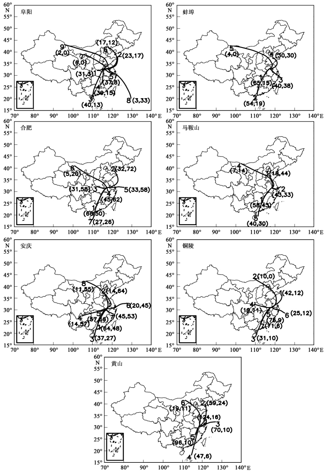
图 4 各观测站 2006 ~ 2008 年降水日 48 h 后向轨迹各组内平均轨迹分布及酸雨观测次数 (括号内左边数字) 和 中度以上酸雨频率 (%) 括号内右边数字)
