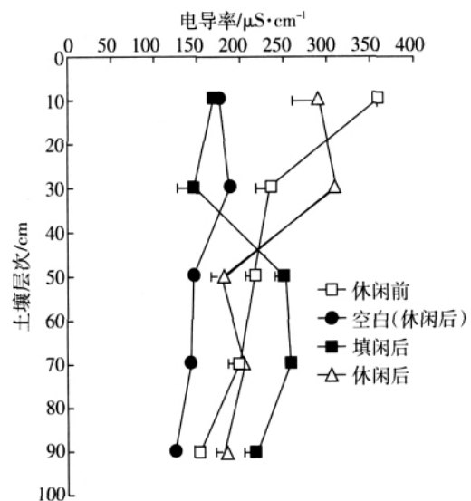
图 5 填闲前后土壤剖面电导率变化
