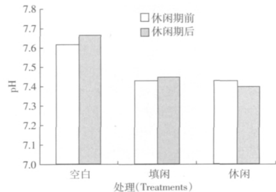
图 4 填闲作物种植前后土壤 pH 变化情况
