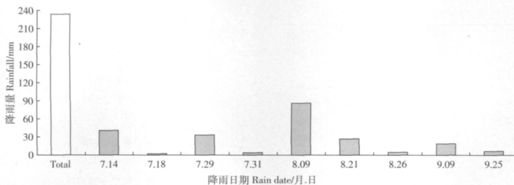
图2 休闲期间降雨量统计
