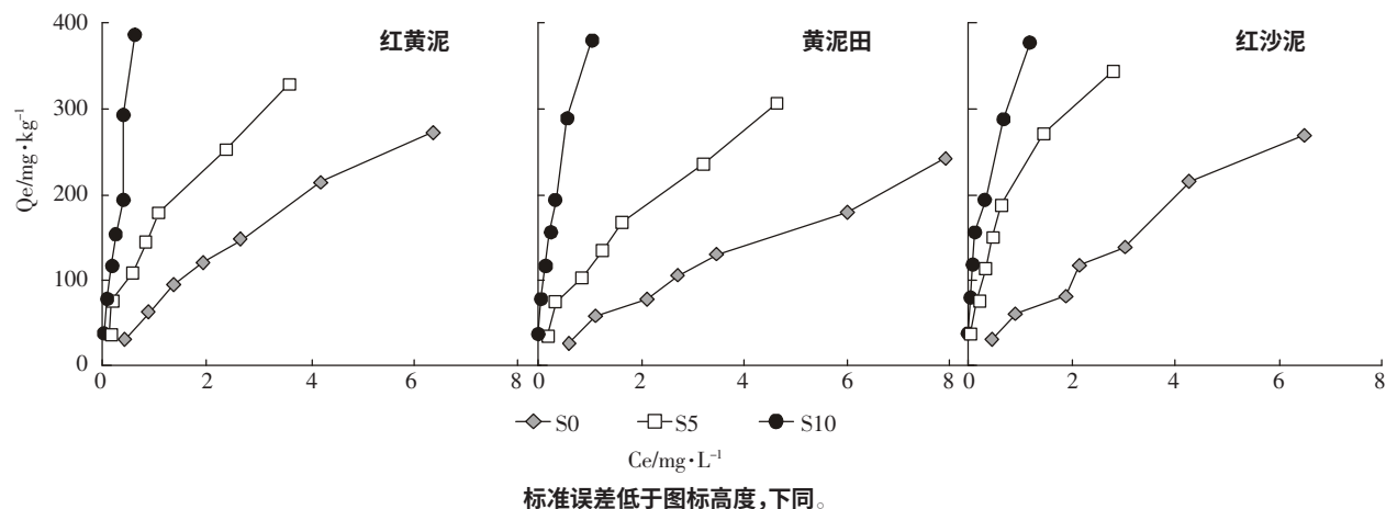
图 1 海泡石对典型水稻土吸附镉的影响
