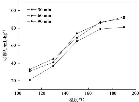
图 3 不同加热时间下可浮油随温度变化
