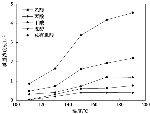
图 2 水热产物有机酸浓度随温度变化
