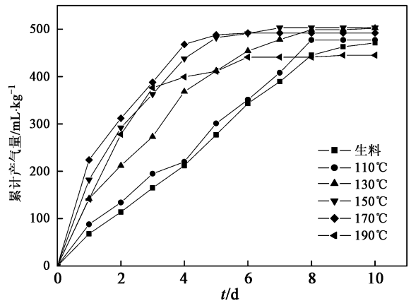
图 4 不同预处理温度下累积比生物气产量变化曲线
