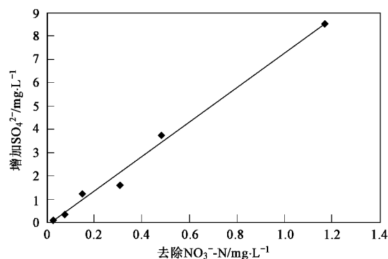
图 4 \text{NO}_3^- -N 去除量与 \text{SO}_4^{2-} 生成量关系曲线
