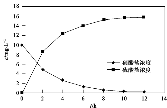
图 3 \text{NO}_3^- 、 \text{SO}_4^{2-} 浓度变化曲线
