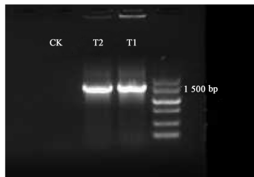
图 6 16S rDNA 全长扩增
