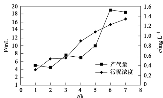
图 1 污泥产气量和浓度变化曲线
