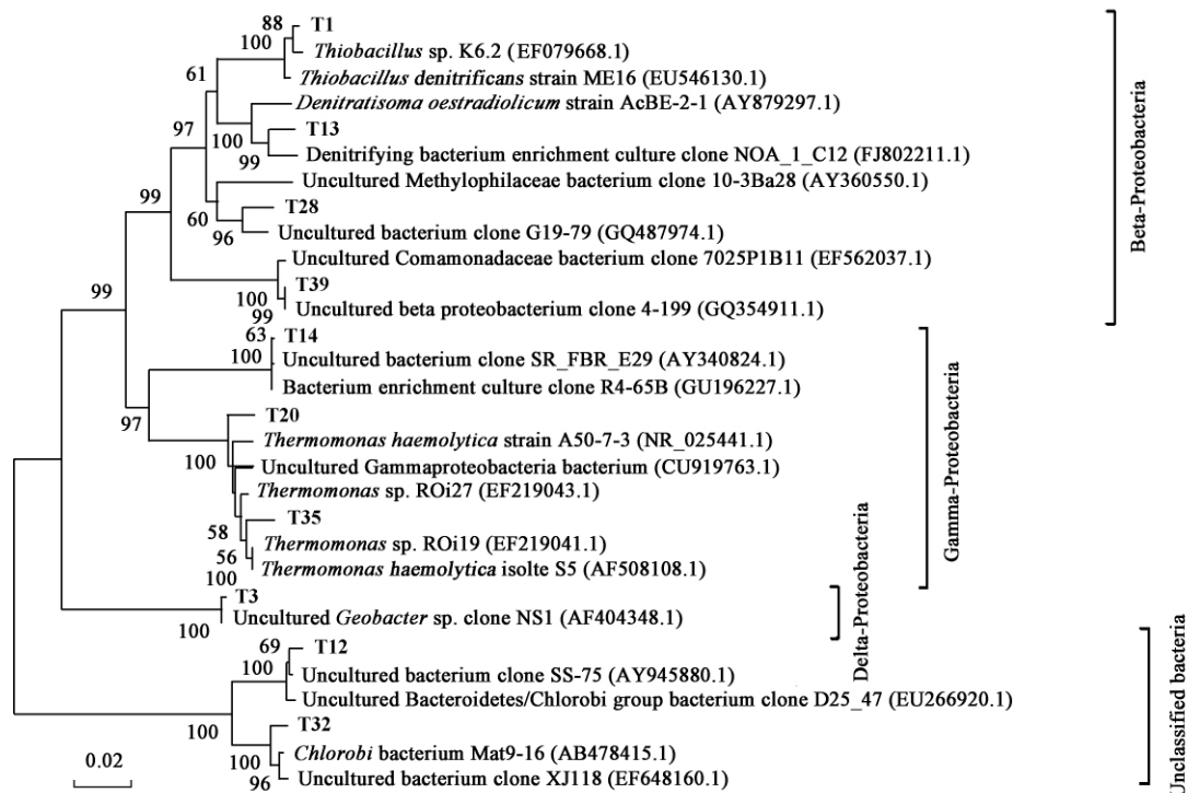
图 8 基于 16S rDNA 序列的细菌系统发育树
