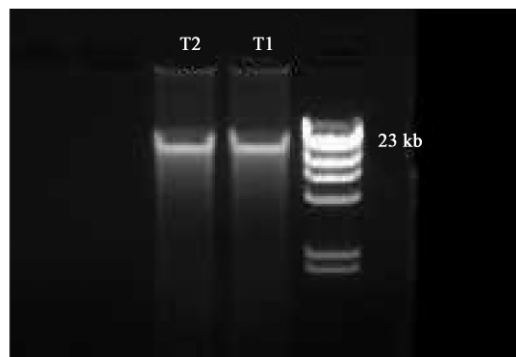
图 5 总 DNA 提取结果
