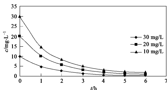
图 2 硝酸盐浓度变化曲线
