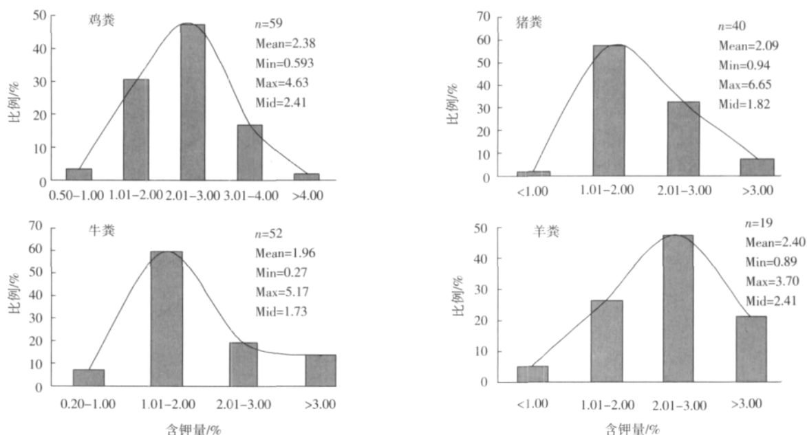
图 3 畜禽粪便中钾素含量的分布状况
