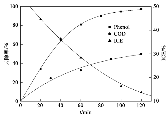
图 5 苯酚和 COD 去除率及电流效率随反应时间的变化
