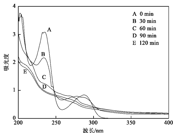
图 4 不同电解时间条件下苯酚的紫外扫描图
