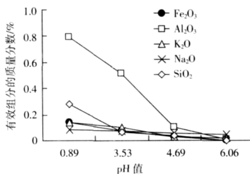
图 5 样品 2 有效元素不同 pH 值下的变化(2)
