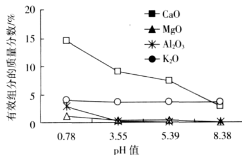
图 6 样品 3 有效元素不同 pH 下的变化(1)
