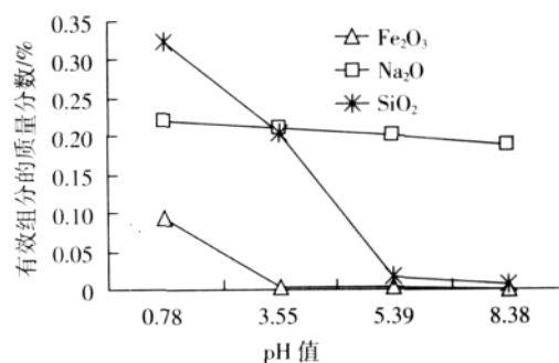
图 7 样品 3 有效元素不同 pH 值下的变化(2)
