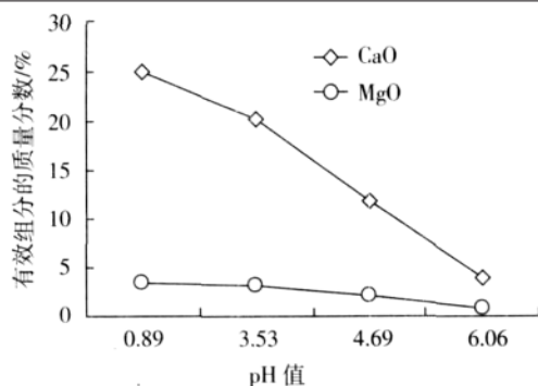
图 4 样品 2 有效元素不同 pH 值下的变化(1)
