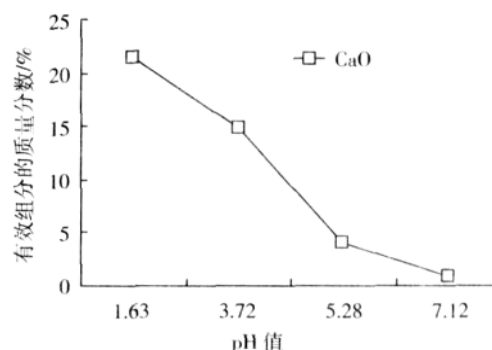
图 2 样品 1 有效元素不同 pH 值下的变化 (1)
