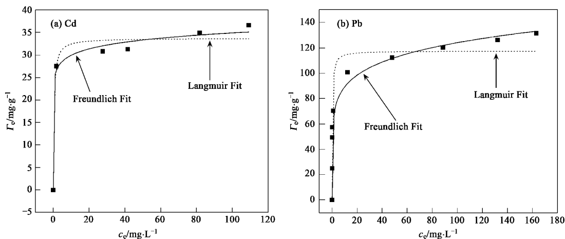
图4 杂化材料对镉和铅的吸附等温线
