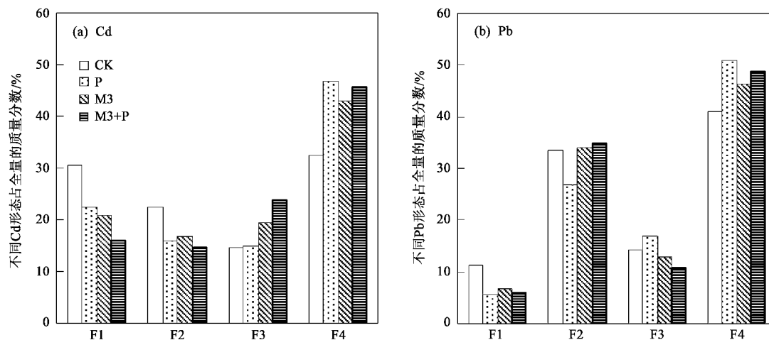
图3 不同杂化材料处理对土壤重金属形态转化的影响
