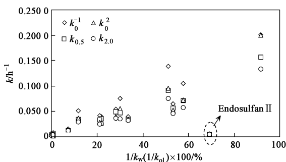
图 2 水相阻力占总交换阻力百分数与挥发速率常数之间的关系
