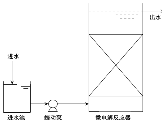
图 1 铁碳微电解实验装置示意
