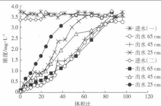
图 10 不同水力负荷下的穿透曲线图
