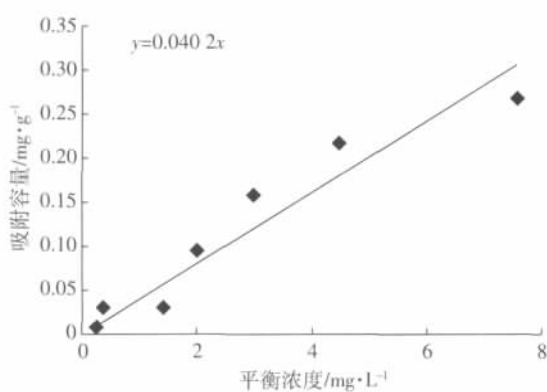
图13 两次再生沸石吸附等温线
