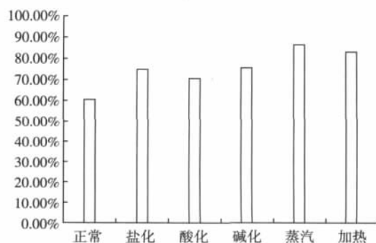
图7 不同活化方法对沸石吸附 \text{NH}_4^+\text{-N} 的影响
