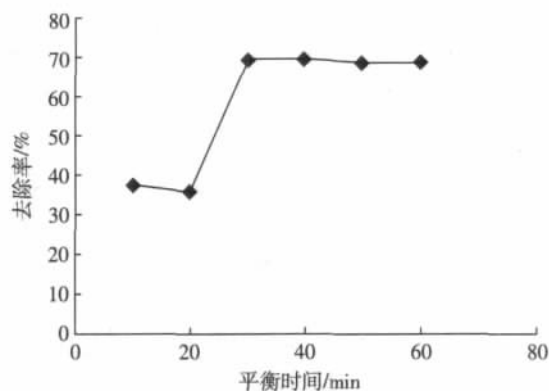
图 1 沸石对 \text{NH}_4^+-\text{N} 的吸附平衡时间关系
