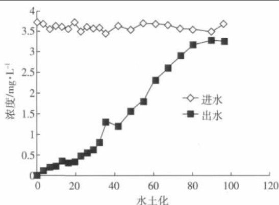
图 8 沸石渗滤床穿透曲线图
