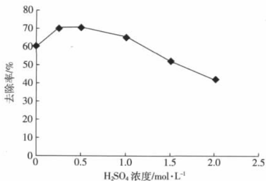
图4 \text{H}_2\text{SO}_4 溶液活化沸石吸附 \text{NH}_4^+\text{-N} 的效果
