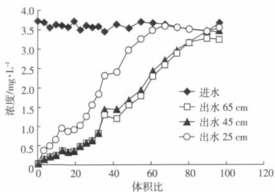
图 9 沸石渗滤床处理效果沿程变化图
