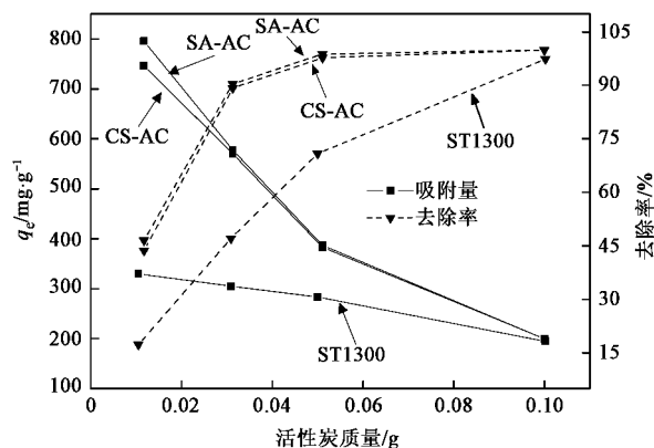
图3 吸附剂量对活性炭对对硝基苯胺的影响
