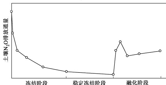
图 1 冻融过程土壤 N_2O 排放特征
