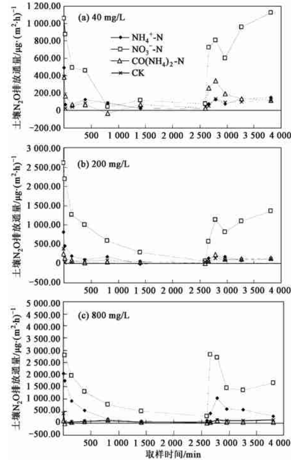
图 2 氮素形态对冻融过程中土壤 N 2 O 排放通量的影响
