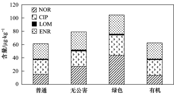
图 5 不同品级蔬菜中喹诺酮类抗生素组成特征 Fig. 5 Constitute of \sum QNs in different levels of vegetable
