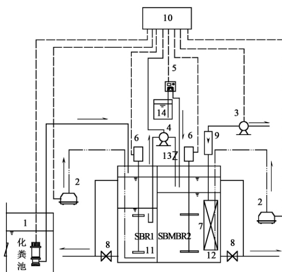
1. 潜污泵; 2. 风机; 3. 抽滤泵; 4. 自吸泵; 5. 蠕动泵; 6. 搅拌电机; 7. 平板膜组件; 8. 放空阀; 9. 流量计; 10. PLC; 11. 微孔曝气管; 12. 穿孔曝气管; 13. 止回阀; 14. 加药桶
