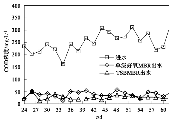
图5 COD 处理效果
