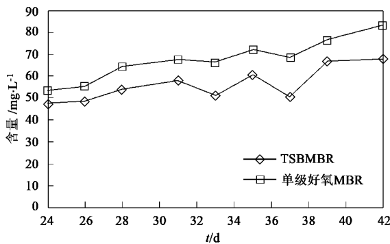
图 9 混合液中 EPS 的变化
