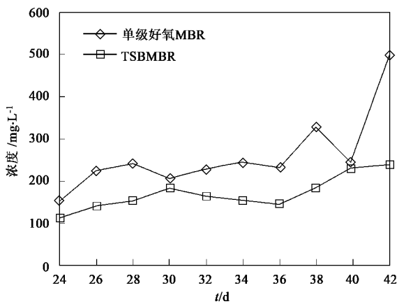
图 8 上清液中 SMP 的变化
