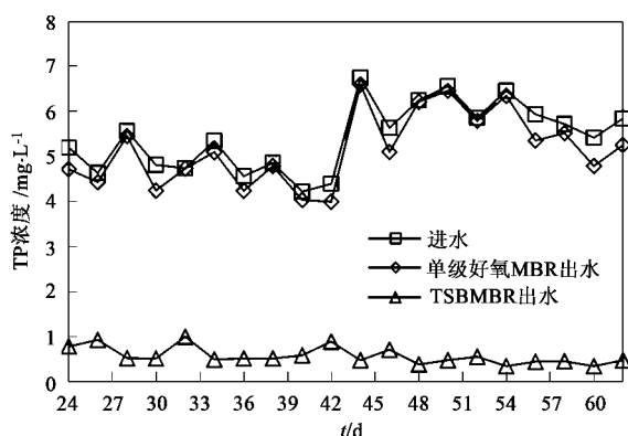
图2 TP 处理效果
