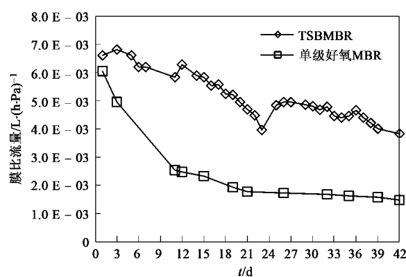
图7 膜比流量的变化
