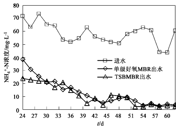
图4 \text{NH}_4^+-\text{N} 处理效果
