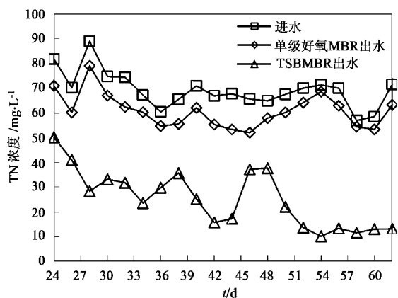
图3 TN 处理效果
