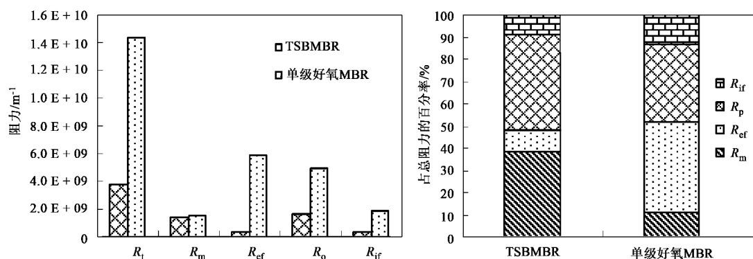
图6 平板膜污染阻力分布
