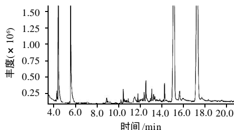
图 1 油菜花中挥发油成分的总离子流图
