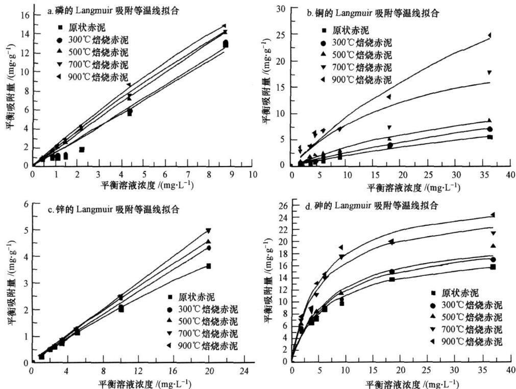
图 1 不同活化方法的吸附剂吸附磷、铜、锌、砷 Langmuir等温吸附曲线拟合
