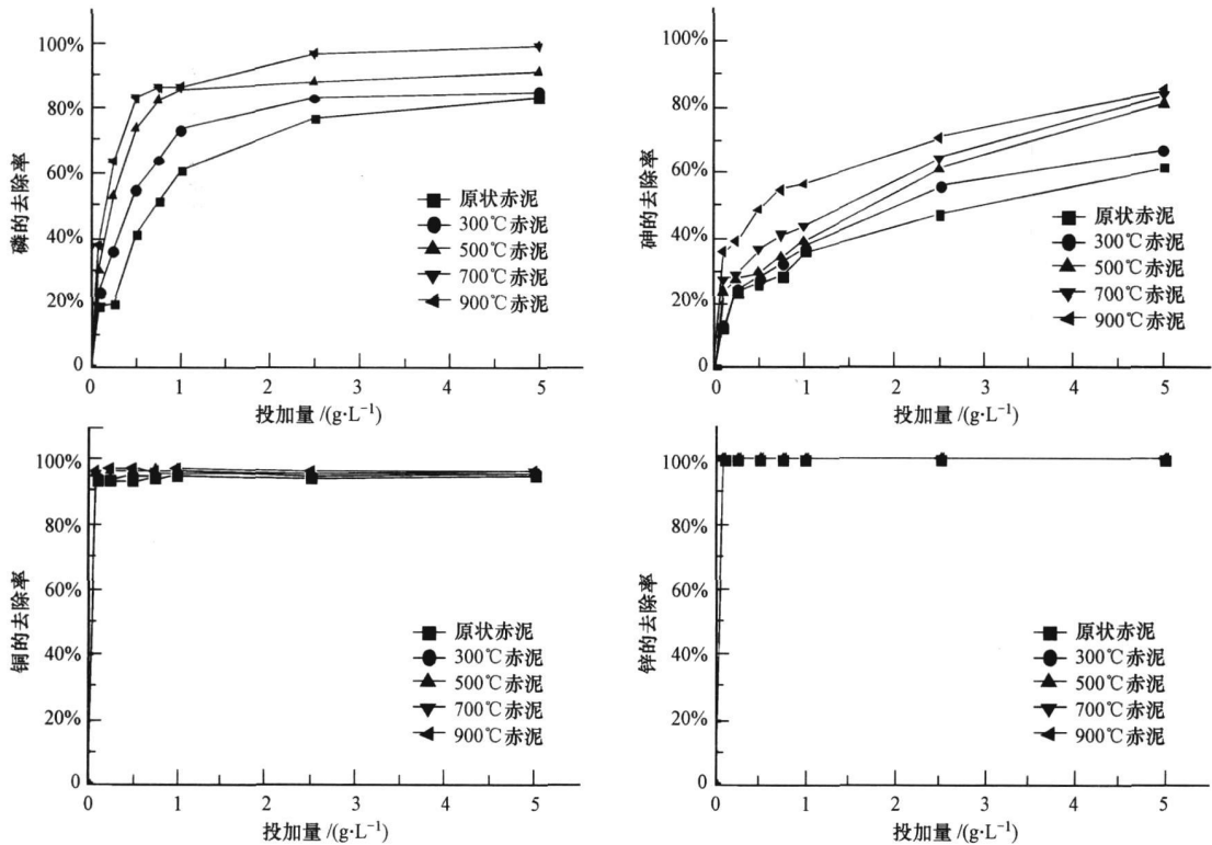
图 2 不同焙烧温度下活化赤泥对畜禽养殖废水 SBR 出水磷、砷、铜、锌的去除率
