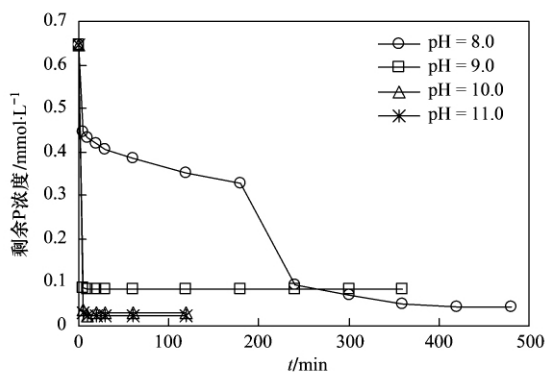
图 2 不同 pH 值下磷浓度随反应时间的变化
