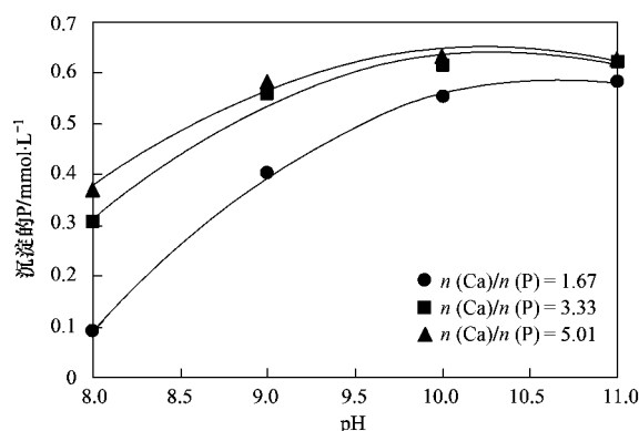
图 3 不同初始 n(\text{Ca})/n(\text{P}) 、不同 pH 值条件下磷的沉淀量
