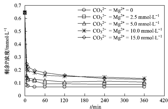
图 8 \text{CO}_3^{2-} 和 \text{Mg}^{2+} 共存对磷酸钙沉淀反应的影响
