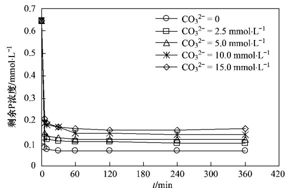
图 4 不同 \text{CO}_3^{2-} 浓度对磷去除的影响
