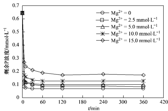
图 6 不同 \text{Mg}^{2+} 浓度对磷去除的影响 Fig. 6 Effects of \text{Mg}^{2+} concentration on phosphate removal
