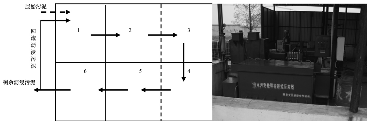
相邻区域隔板实线表示隔板露出水面, 底部向上 1/4 高度区间为污泥流过通道; 虚线表示隔板位于水下, 从水面向下 1/4 区间为污泥流过通道
