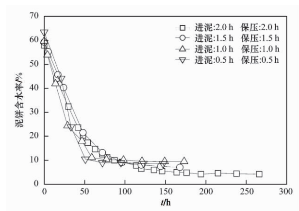
图 5 不同压滤时间脱水泥饼的水分蒸发情况(25℃)
