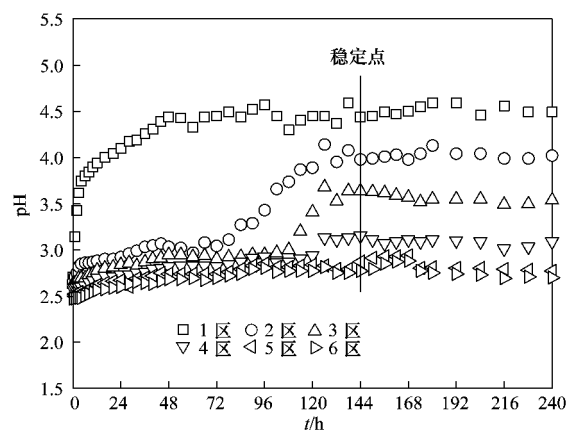
图 2 推流式生物沥浸反应器系统污泥 pH 随时间的变化
