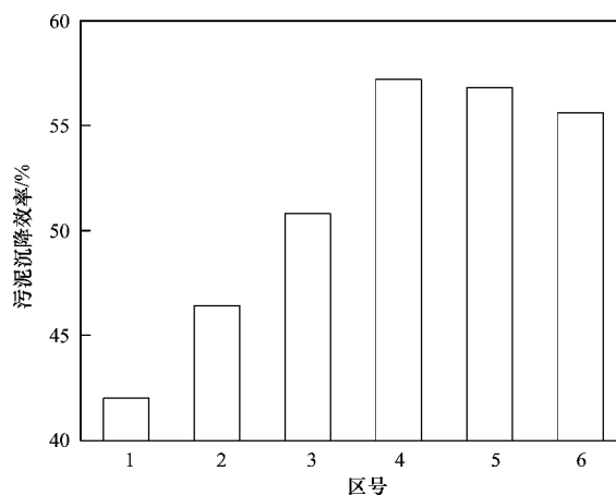
图4 反应器达到稳态时各区污泥的沉降效率
