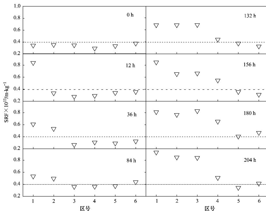
图3 推流式生物沥浸反应器系统各区污泥比阻值随时间的变化
