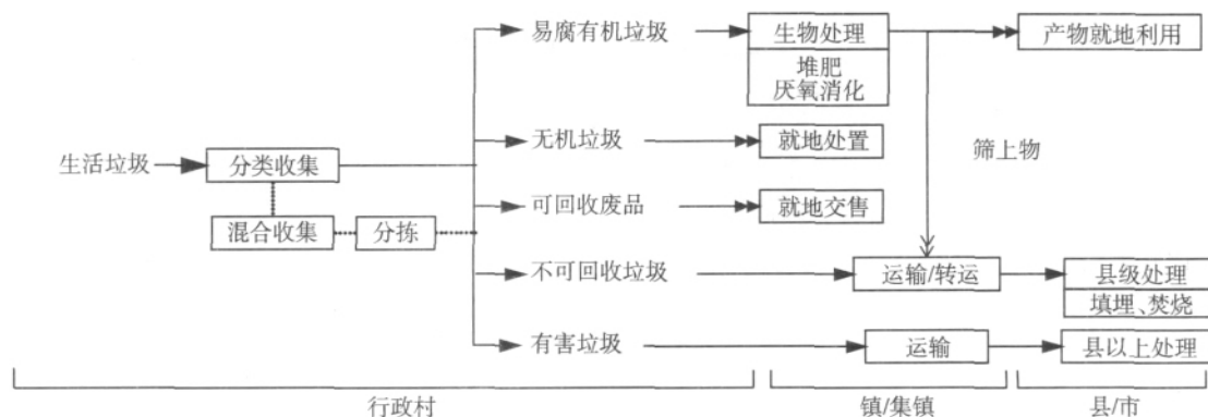
图1 基于分类处理的村镇生活垃圾处理技术路线
