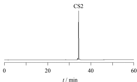
图5 Fr. 6 中组分 2 的 HPLC 色谱图
