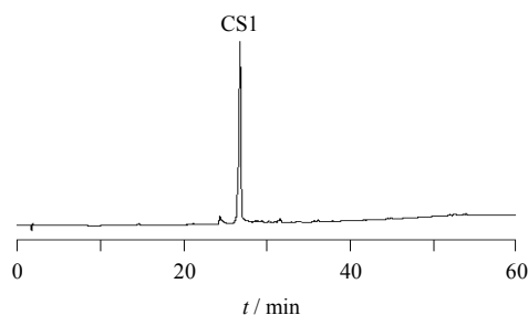
图3 Fr. 4 中组分 3 的 HPLC 色谱图
