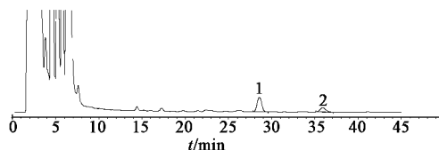
图3 传统汤剂图
