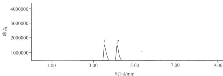
图 1 甲醇和苯的色谱图
