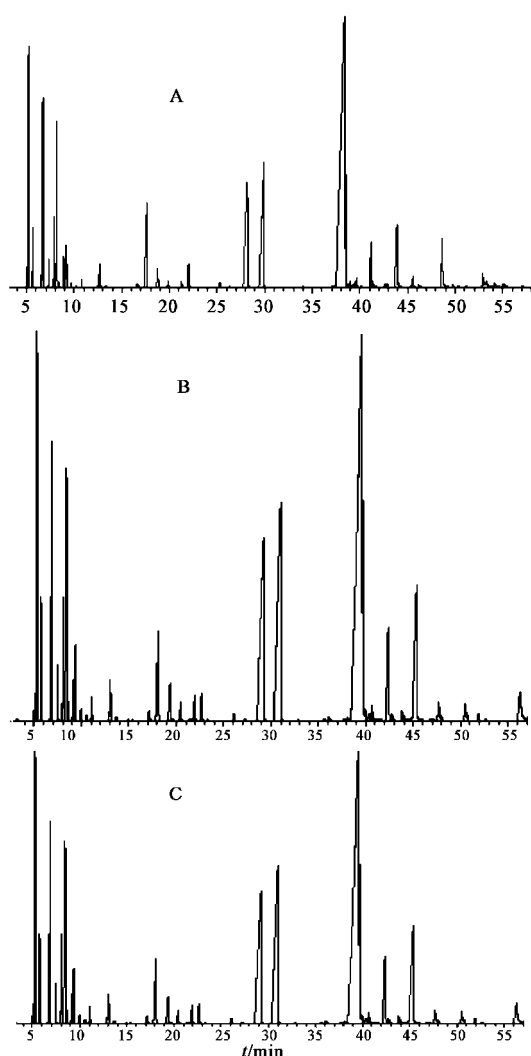
图1 3种细辛挥发性成分的总离子流色谱图 A. 黑龙江产; B. 辽宁产; C. 吉林产
