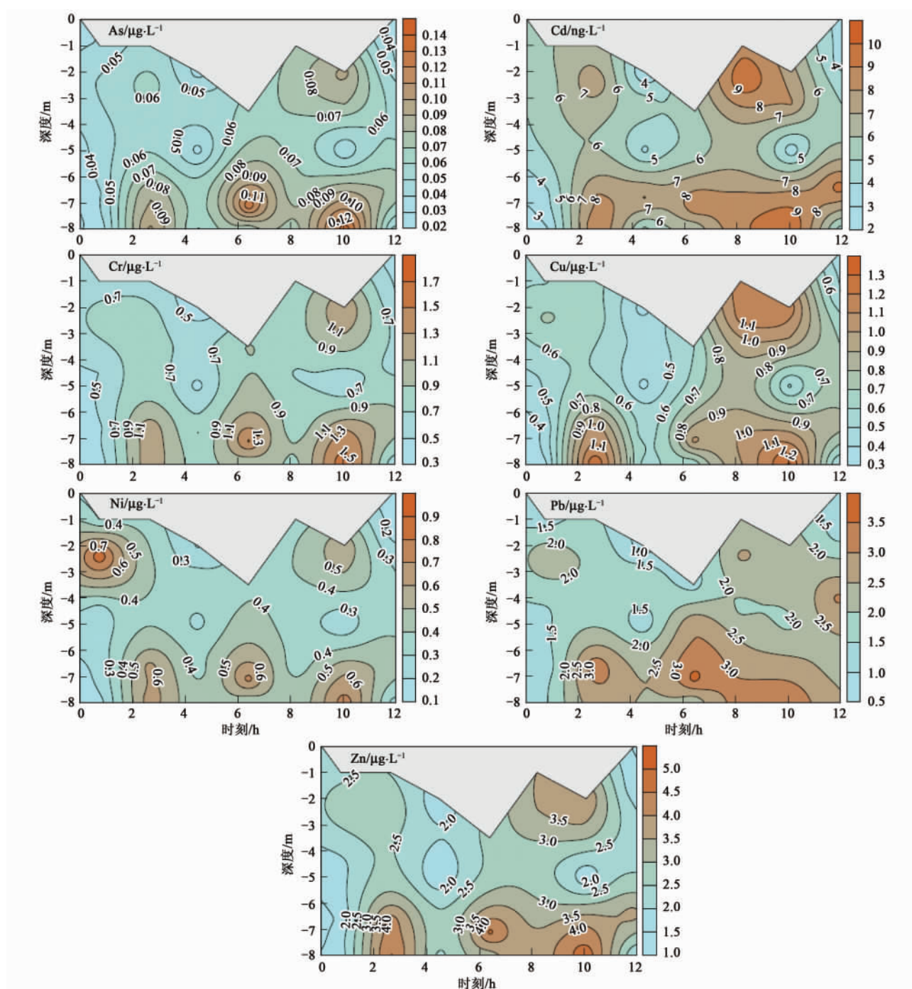
图3 Q2站悬浮颗粒物中重金属分布
