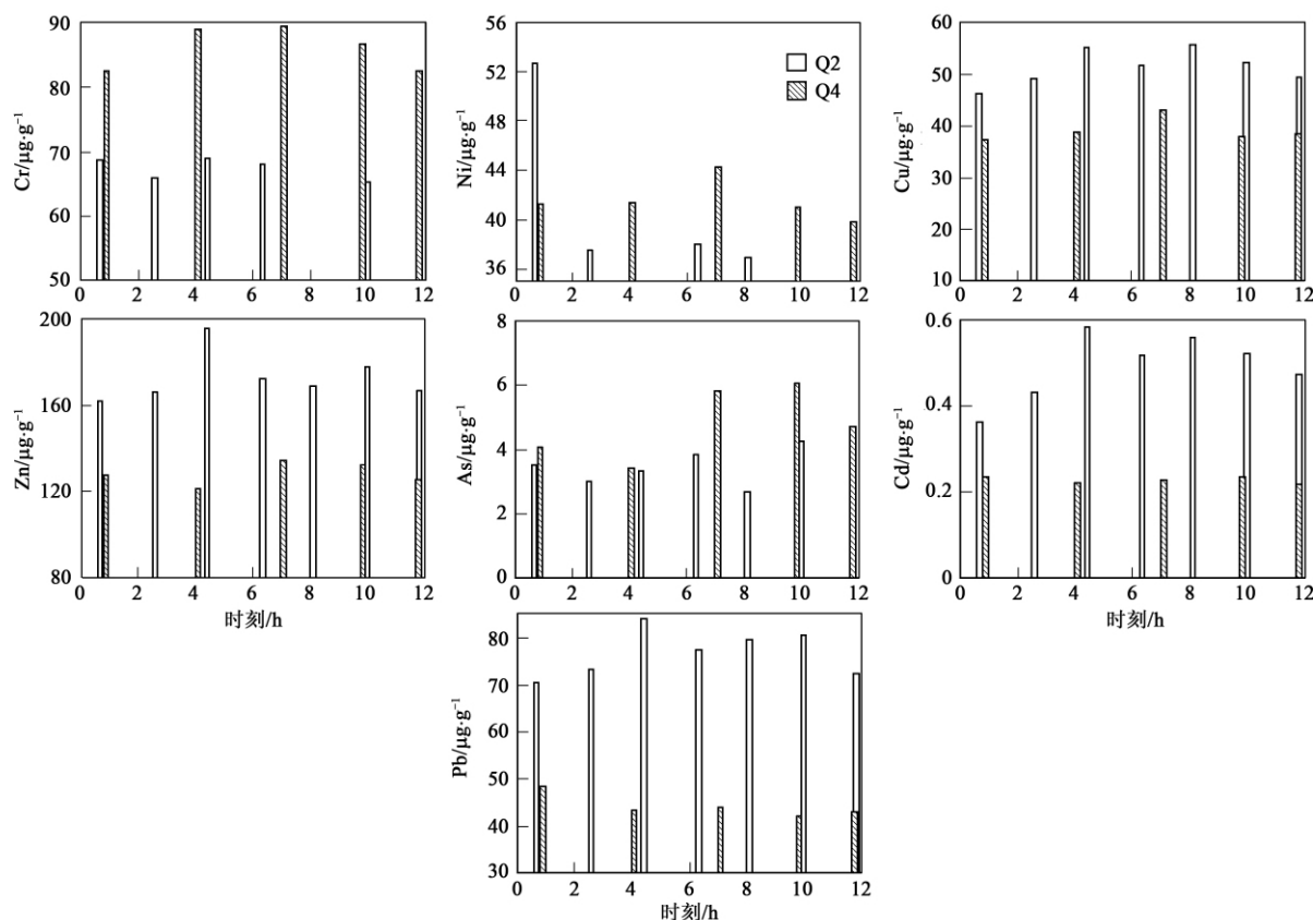
图 5 Q2、Q4 站表层沉积物中重金属分布
