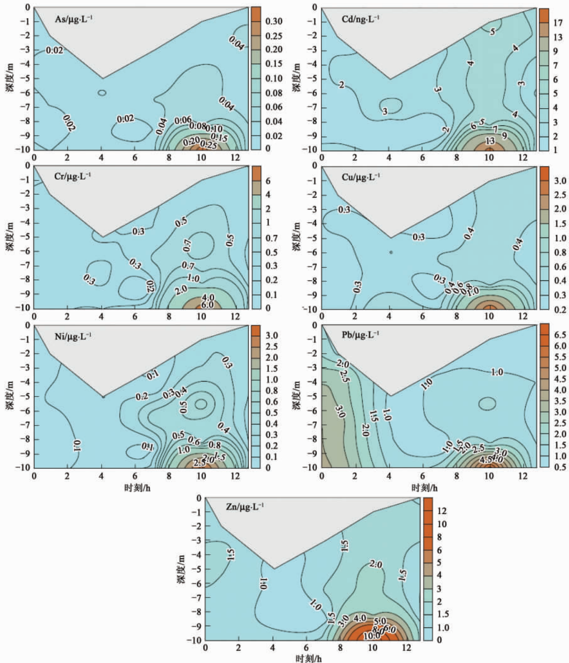
图 4 Q4 站悬浮颗粒物中重金属分布
