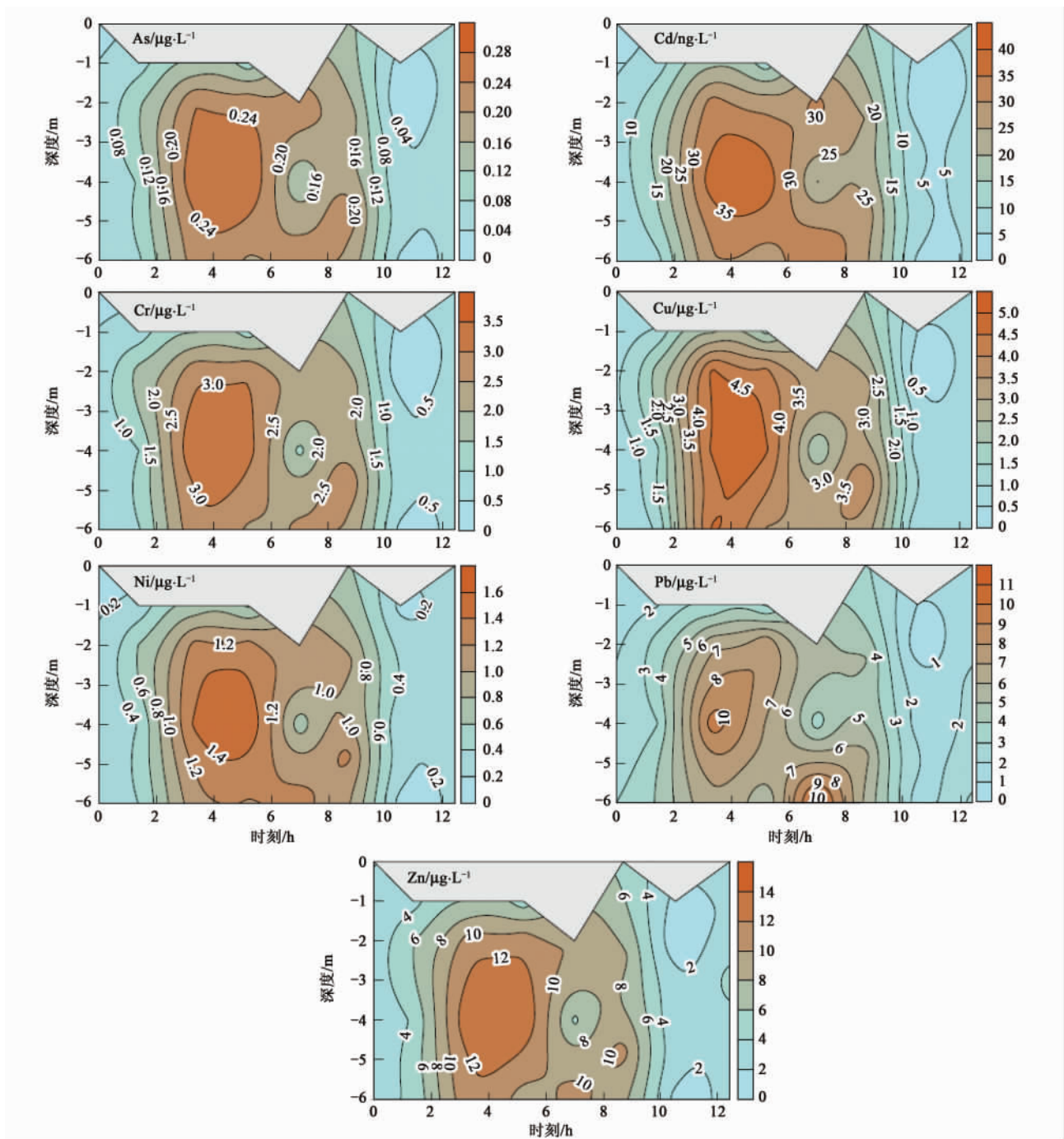
图2 Q1 站悬浮颗粒物中重金属分布
