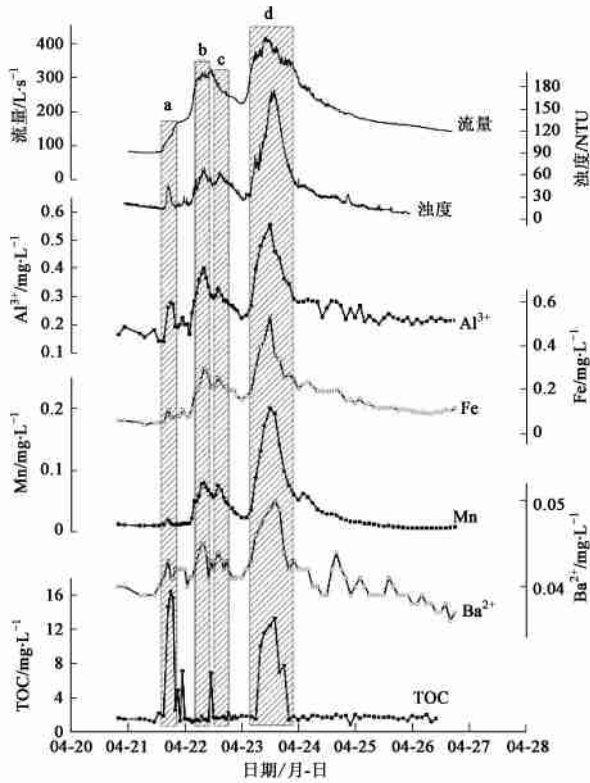
图3 2008年4月下旬姜家泉泉水中部分阳离子、TOC浓度变化
