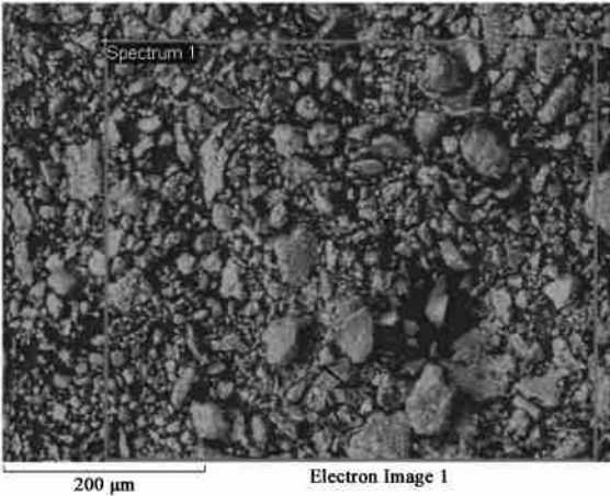
图4 c阶段姜家泉泉水中悬浮颗粒物SEM和EDS图
