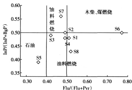
图 2 天津大沽排水河沉积物 \text{InP}/(\text{InP}+\text{BgP}) 和 \text{Flu}/(\text{Flu}+\text{Pyr}) 值散点图
