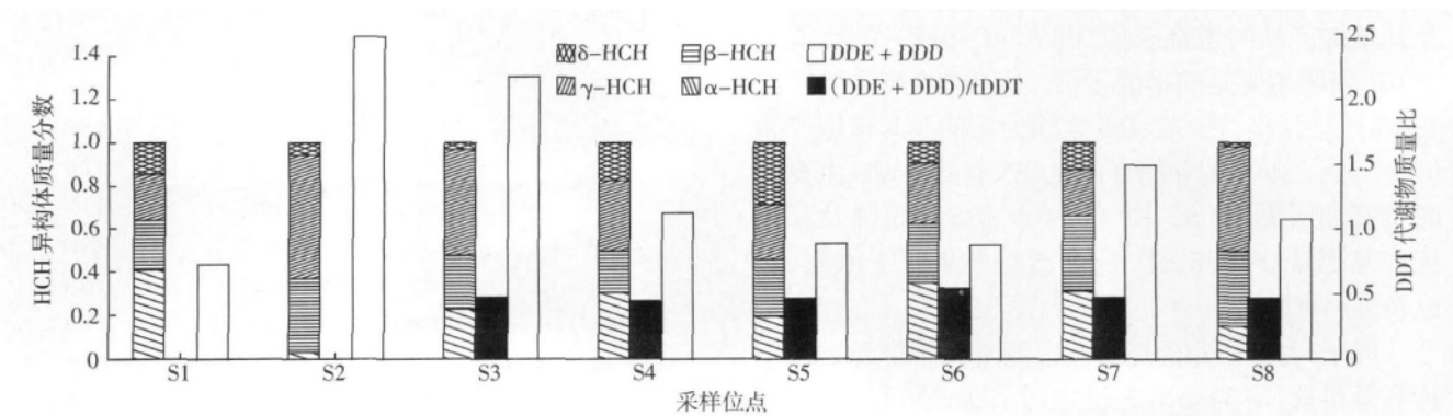
图 3 大沽排水河沉积物 HCH 异构体组成比及 DDD/DDE 和 (DDD+DDE)/tDDT 比值
