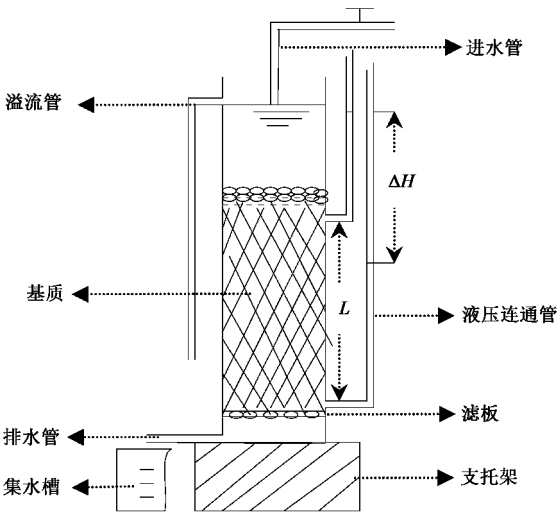
图 1 常水头渗透试验装置 Fig. 1 Device of ordinary water experiment
