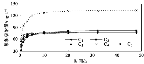
图 4 TP 的静态累积吸附量
