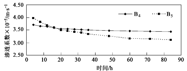
图 6 2 种基质的污水渗透系数
