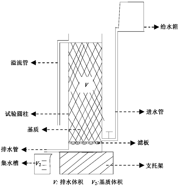
图 2 给水度试验装置 Fig. 2 Device of feed water experiment
