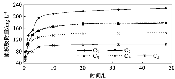
图 3 TN 的静态累积吸附量
