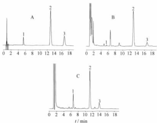
A. 对照品; B. 样品(本文色谱条件); C. (药典色谱条件); 1. 柠檬苦素; 2. 吴茱萸碱; 3. 吴茱萸次碱。 图 1 不同色谱条件下的 HPLC 图
