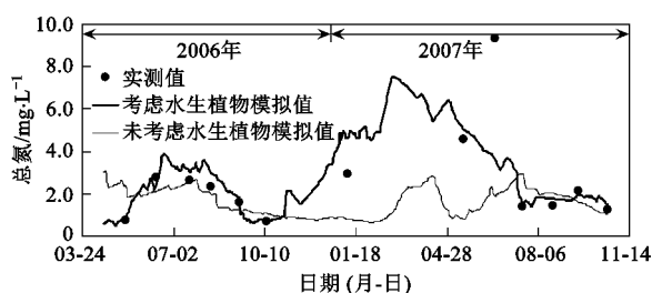
图2 挺水植物对总氮模拟结果的影响
