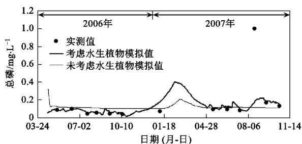
图5 挺水植物对总磷模拟结果的影响
