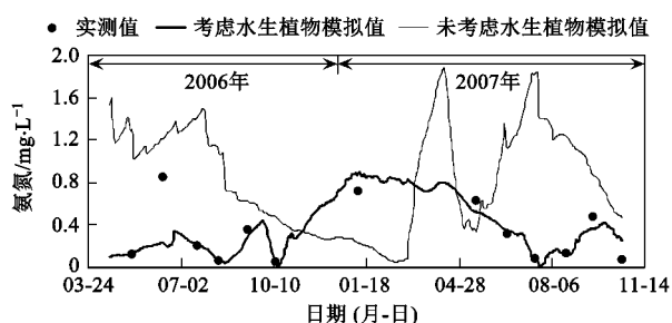
图3 挺水植物对氨氮模拟结果的影响
