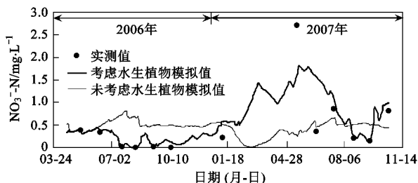
图4 挺水植物对硝态氮模拟结果的影响
