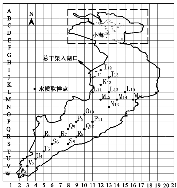
图1 乌梁素海水质监测点分布示意
