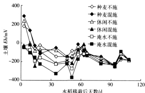
图 2 土壤 E_h 的季节变化 Figure 2 Seasonal variation of soil E_h
