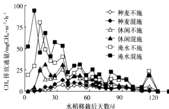
图 1 CH 4 排放通量的季节变化
