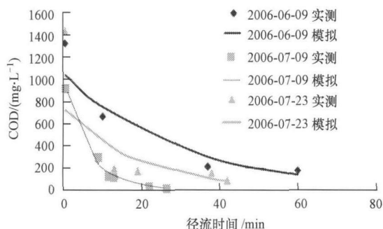
图 2 屋面雨水水质变化过程 (潘国庆, 2007)
