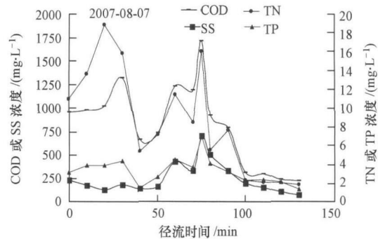
图 4 某道路雨水干管次降雨水质变化过程
