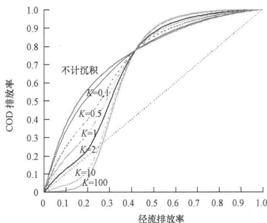
图 5 管道沉积物对初期冲刷效应的影响
