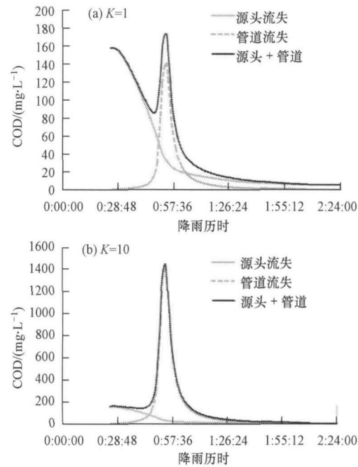
图 3 管道沉积物对浓度变化过程的影响
