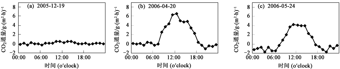
图 3 农田 CO 2 通量的典型日变化过程比较
