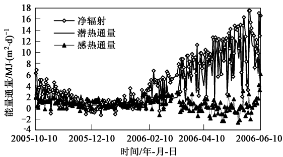
图 2 农田能量通量日际变化曲线
