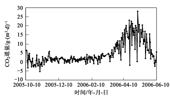
图 4 农田 CO 2 通量日际变化曲线
