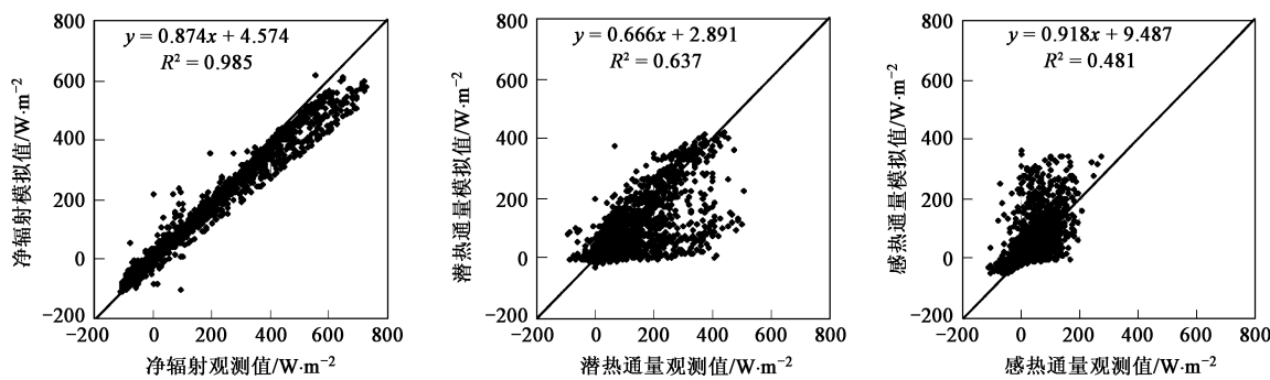
图 5 农田净辐射、潜热通量及感热通量模拟值与观测值对比
