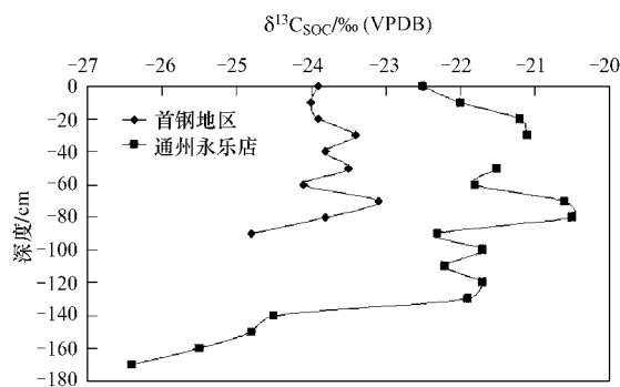
图 1 北京地区土壤剖面有机碳同位素组成
