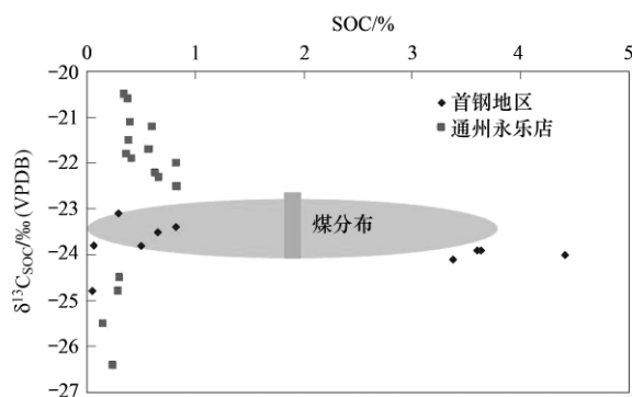
图3 北京地区土壤样品(本研究)和中国煤 [18] 的 \delta^{13}\text{C}_{\text{SOC}} 和SOC对比图
