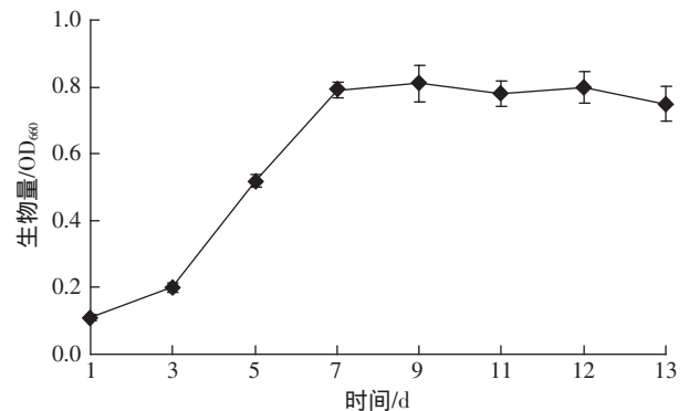
图 1 复合菌群的生物量
