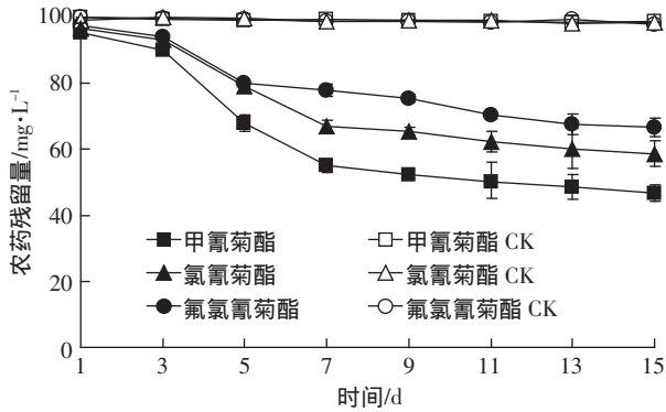
图 2 复合菌群 JZ-1 降解拟除虫菊酯农药效率
