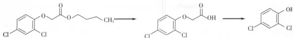
图3 2,4-D 丁酯的主要水解途径
