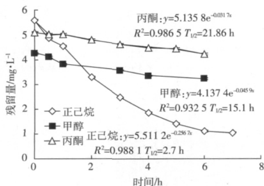
图4 2,4-D 丁酯在正己烷, 甲醇和丙酮中的光解
