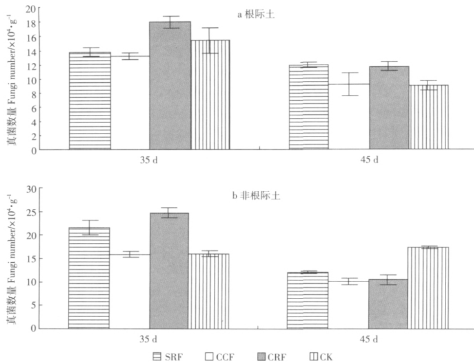
图4 酸性菜园土壤真菌数量
