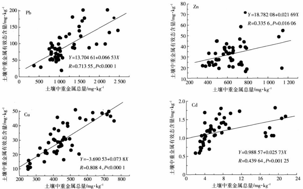
图 1 土壤重金属 DTPA 提取态与总量相关性分析(n=51)
