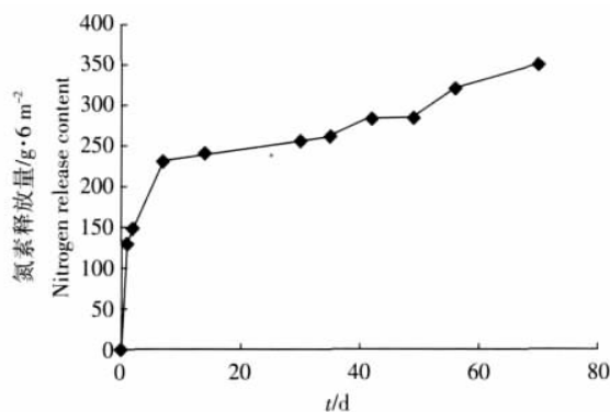
图 1 包膜尿素养分释放量曲线
